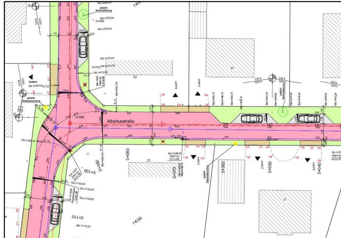
Ausschnitt Ausführungszeichnung „Albartusstraße“
